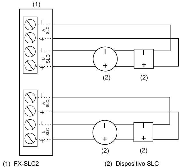
Figura 5: Cableado Clase A [1]
