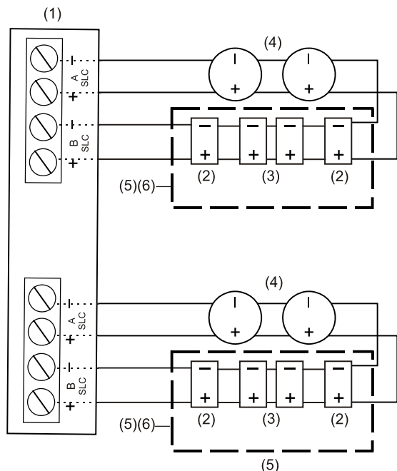
Figura 6: Cableado Clase X [2]
